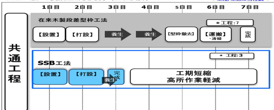
SSB工法PC裏段差部使用例（自社試算）
